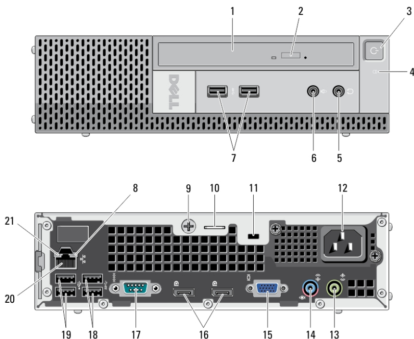
Obrázok 5. Pohľad spredu a zozadu na model Ultra Small Form Factor
